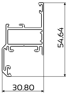
DIE No. W57496 Cas28 Sash Euro
