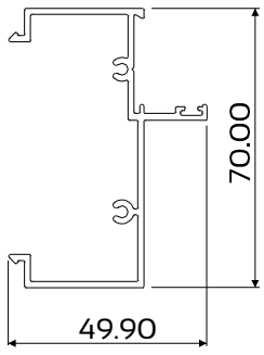
DIE No. W70963 Cas28 Frame 70mm
