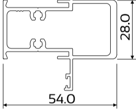
DIE No. W56269 Cas34 54mm Mullion
