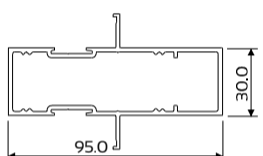
DIE No. W44090 Mullion W95
