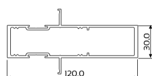
DIE No. W44092 Mullion W120
