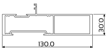
DIE No. W56334
