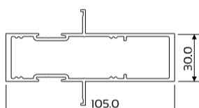
DIE No. W44091 Mullion W105
