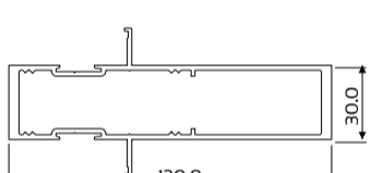
DIE No. W56083 Mullion W130
